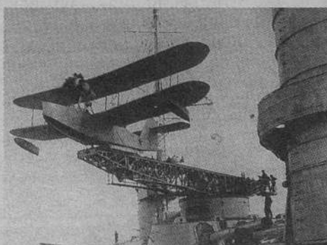
Старт гидросамолета КР-1 («Henkel» HD-55) с катапульты линкора «Парижская коммуна»
